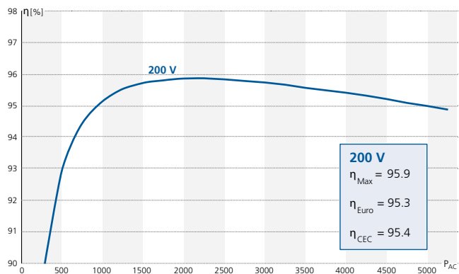
Wirkungsgradkennlinie Powador 6002
