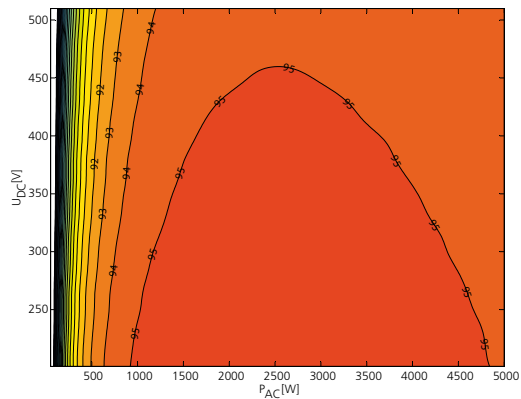
3D-Wirkungsgraddiagramm Powador 6002
